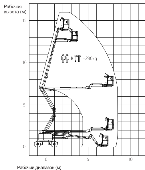
LA14JE Кривая производительности
